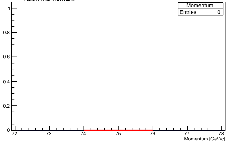
Kaon momentum
