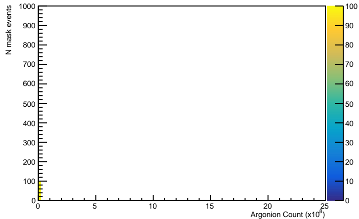
nEventsVsArgonionMask0
