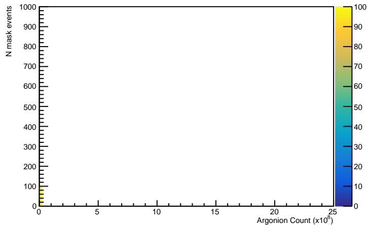
nEventsVsArgonionMask10
