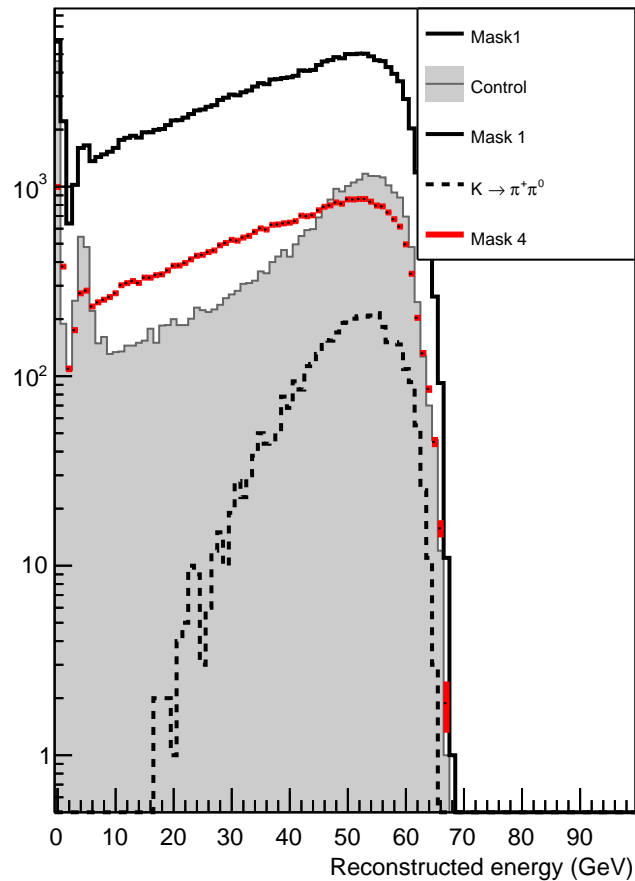
LKrEnergy_C
