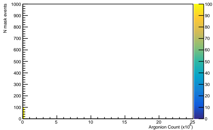
nEventsVsArgonionMask11
