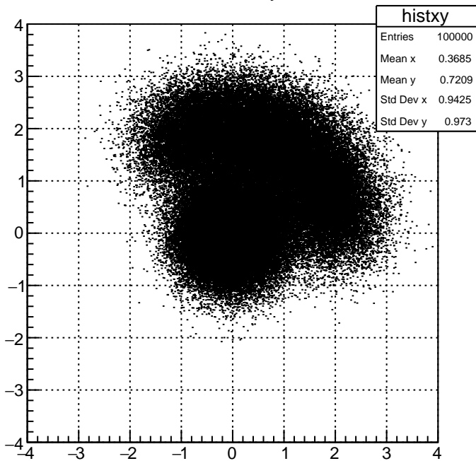
MPL histxy
