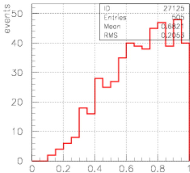
Zp no electron
